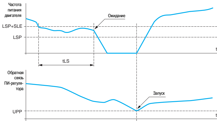
Функции ожидание / запуск
