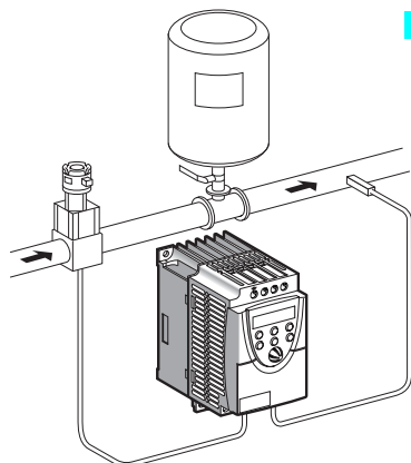
Режим регулирования одной переменной
