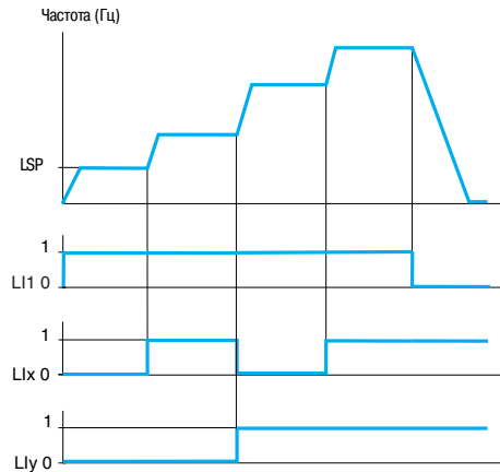
Пример работы с 4 заданными скоростями
