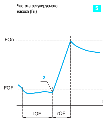
Останов вспомогательного насоса
