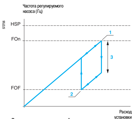
Режим регулирования одной переменной со вспомогательным насосом: гистерезис
