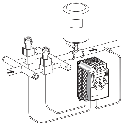
Режим регулирования одной переменной со вспомогательным насосом
