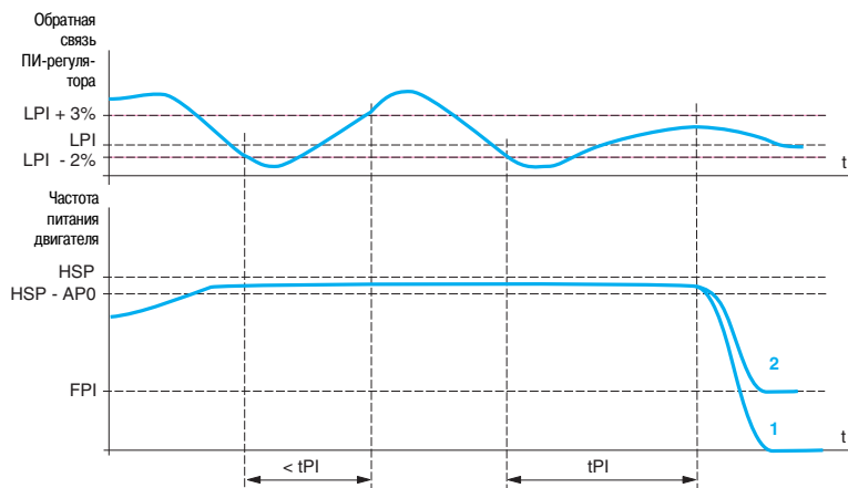
Наблюдение за обратной связью ПИ-регулятора
